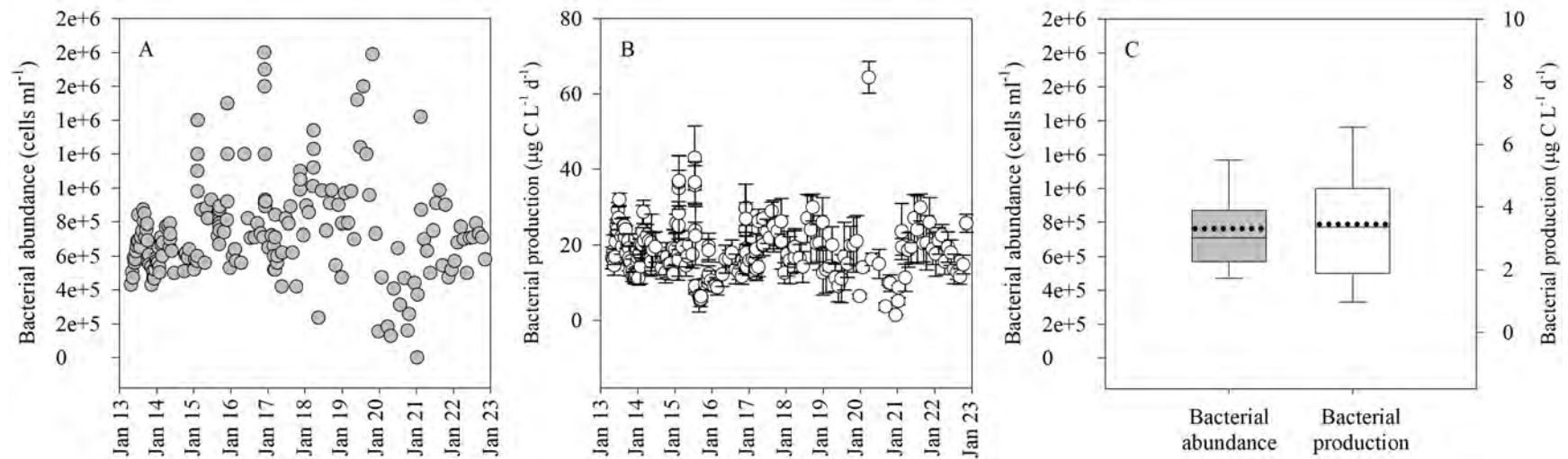
איור 2.1 – שכיחות חיידקים (A) ויצרנות חיידקית (B) בפני השטח (~1 מ') של חוף שקמונה בין השנים 2013 ל 2022. הממוצע הרב שנתי של ערכים אלה מוצג כגרף קופסה (C). הקו בקופסה מייצג את ערך החציון כפי שחושב עבור השנים 2013-2022 בעוד שהקו המקווקו מראה את ערך החציון עבור 2022. שפיעות החיידקים נמדדה בעזרת ציטומטר זרימה וקצבי יצרנות חיידקית נמדדו בעזרת סמן רדיואקטיבי. הדיגום החודשי מאפשר לאמוד את העונתיות החיידקית וקצבי פעילותם במימי חוף שקמונה המוגדרים אוליגוטרופים (עניים בנוטריאנטים), עם ערכים גבוהים בחודשי הקיץ ונמוכים יותר בחורף (פי 1.5), זאת בשונה משכיחות האצות. כמו כן, ניתן לראות חריגות נקודתיות בערכים אלה בעת הזרמת שפכים/גשם/ סופות אבק/זיהום נפט וכד'. בשנת 2022 לא נמצאו חריגות ביחס לממוצע הרב שנתי.
