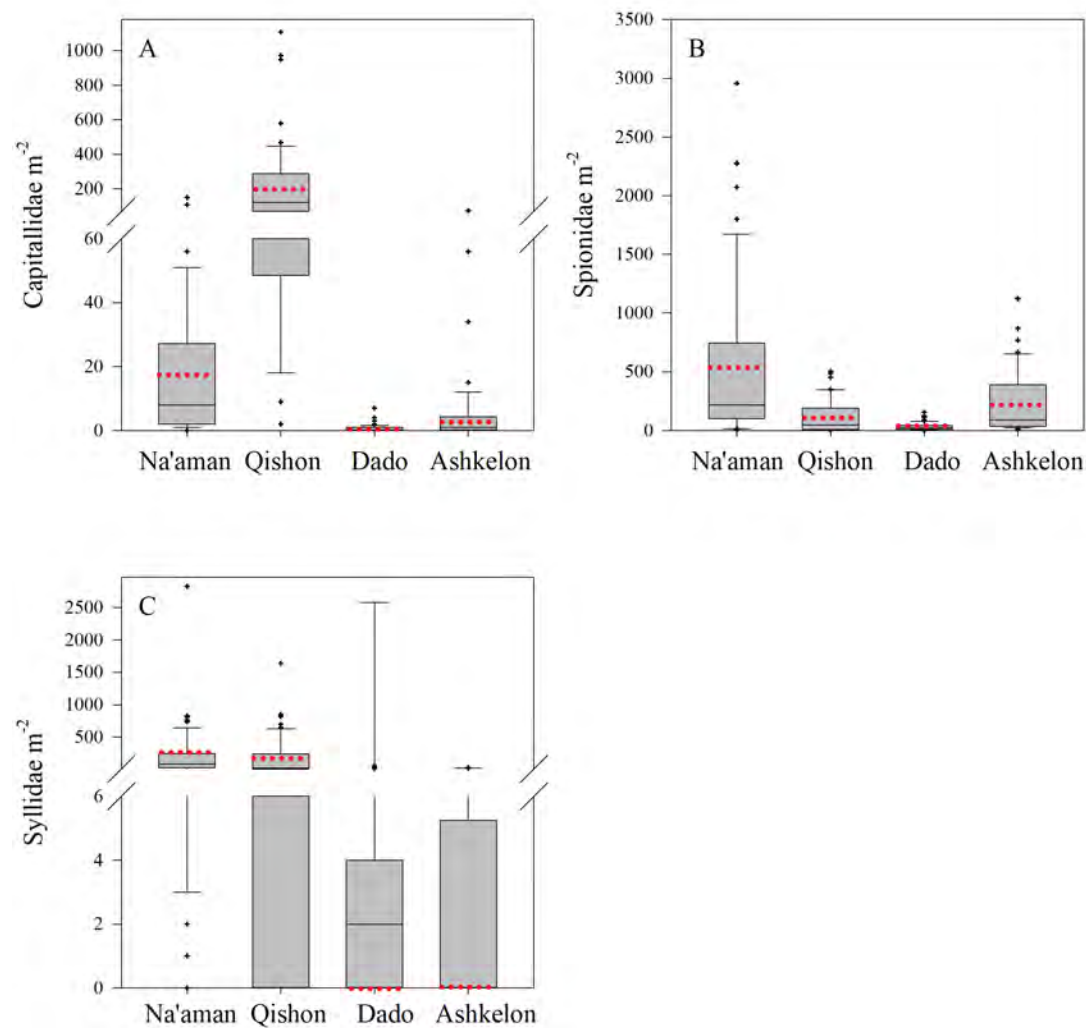
איור 4.7: מספר הפרטים של תולעים רב זיפיות משלושת המשפחות הנפוצות בניטור: Capitalidae (A), Spionidae (B), ו- Syllidae (C) בתחנות נעמן, שפך הקישון, דדו, ואשקלון בין השנים 2005-2022. הקו השחור בתוך הקופסה מייצג את ערך החציון משנות הדיגום. הקו האדום מייצג את ערך הממוצע ב- 2022 (3 חזרות).
