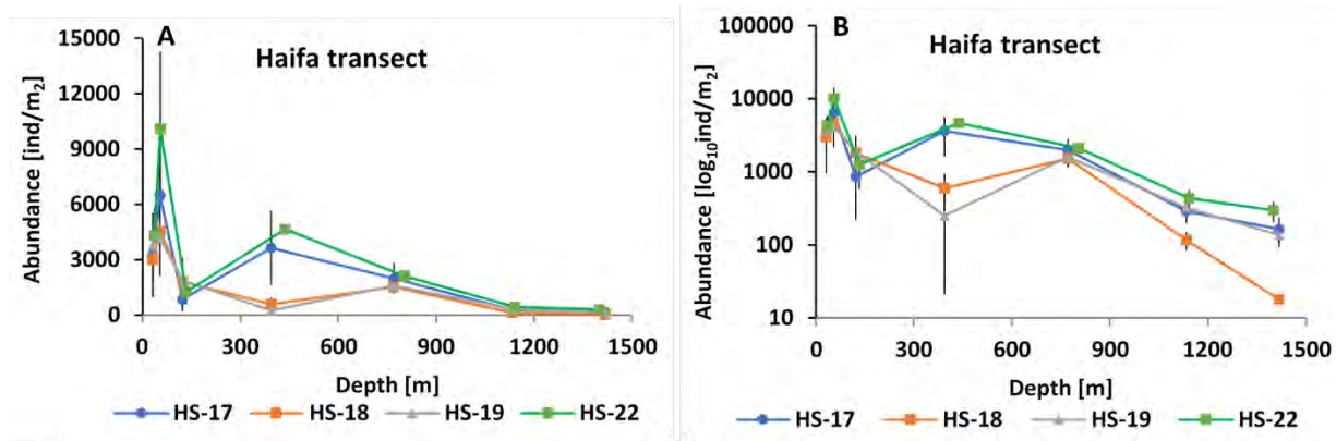
איור 4.11: צפיפות חי תוך המצע, חתך חיפה, בניטורי הים העמוק בשנים 2017-2022. A- סקאלה לינארית. B- סקאלה לוגריתמית.
