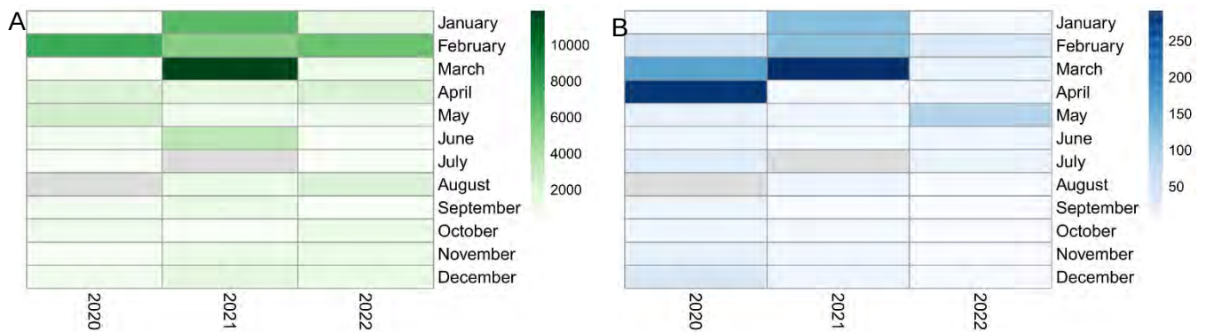
איור 3.7: שכיחות וריכוז ביומסת הזואופלנקטון בתחנת הניטור החופית בחדרה בשנים 2020-2022 - A. שכיחות (מספר פרטים למ"ק) - B. ביומסה (מיליגרם משקל יבש למ"ק).
