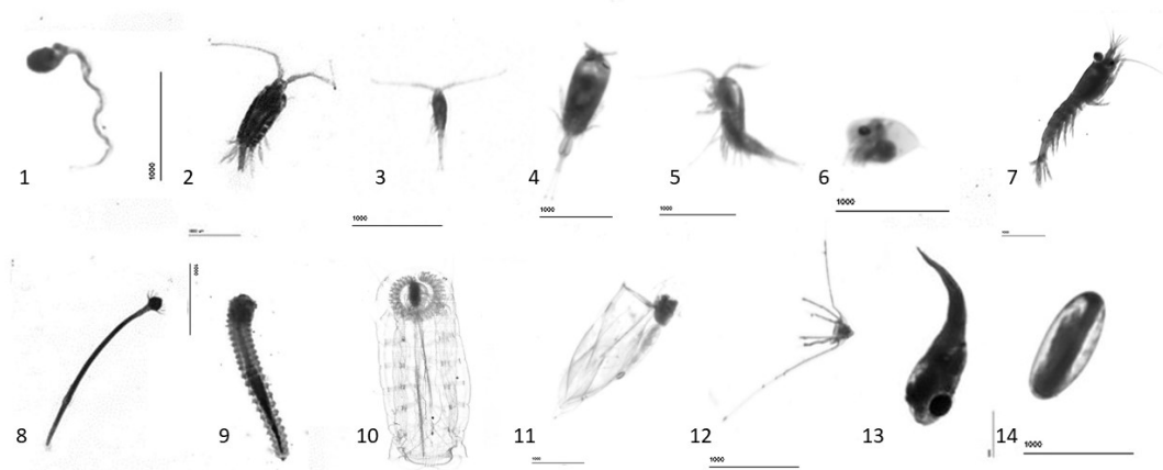
איור 3.4: קבוצות פונקציונליות בזואופלנקטון החופי בתחנת הדיגום החופית בחדרה. A. צלמיות מסריקת הדוגמאות: 1. אפנדיקולריה (Appendicularia), 2. שטרגליים קלנאידים (Calanoida), 3-4. שטרגליים ציקלופואידים (Cyclopoida), 5. שטרגליים הרפקטיקואידים (Harpacticoida), 6. דפניטאיים (Diplostraca), 7. סרטנים מעשירי-רגל (Decapoda), 8. תולעי-חץ (Chaetognatha), 9. תולעים רב-זיפיות (Polychaeta), 10. סאלפות (Salpidae), 11. סיפונופורה (Siphonophorae), 12. קווצי-עור (Echinodermata), 13. לאריות דגים, 14. ביצי דגים. B. שכיחות יחסית (%) של הקבוצות הפונקציונליות לאורך חודשי שנת 2022.
