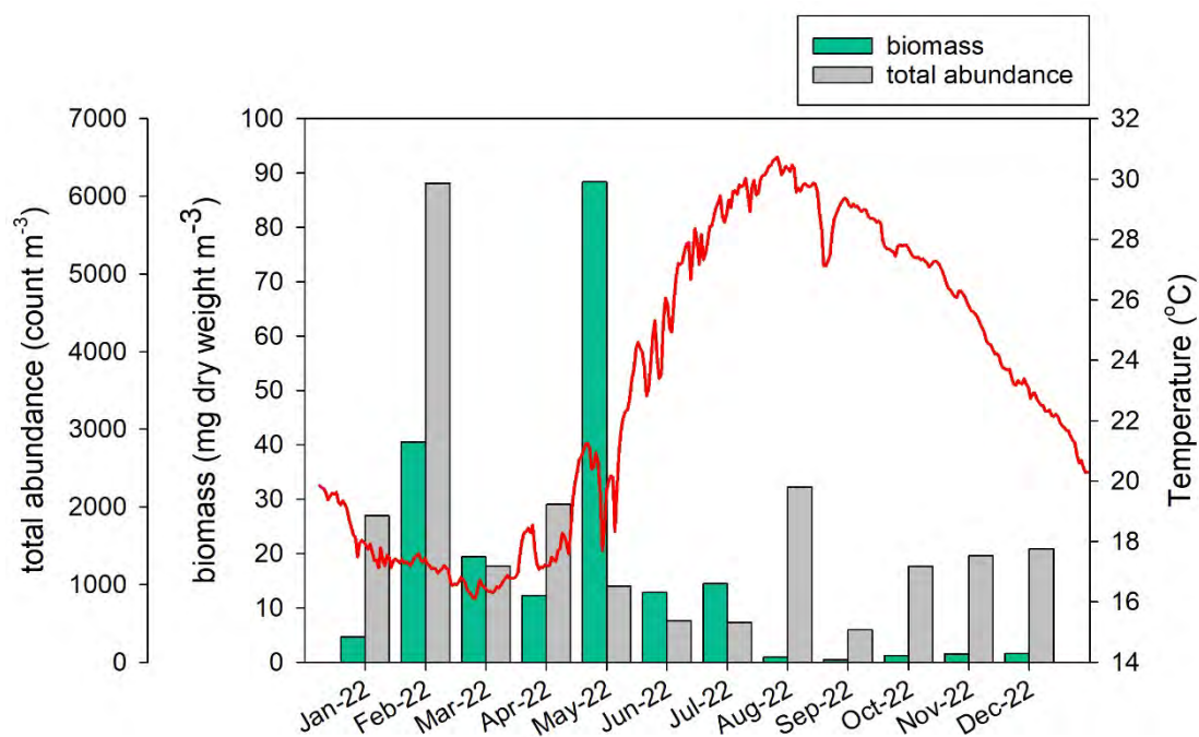
איור 3.3: שכיחות וריכוז ביומסת זואופלנקטון (מספר פרטים ומיליגרם משקל יבש למטר מעוקב, בהתאמה) בגודל < 200 \mu\text{m} בעמודת המים (0-25 מ') במים החופיים בתחנה המטאורימית בחדרה בשנת 2022. הדיגום נערך באמצעות גרירה אנכית של רשת מסוג WP2 (Hydro-Bios) במהירות > 1 \text{ מ'}/\text{שניה} . כמות הפרטים התקבלה ע"י סריקה ממוחשבת של דוגמת הרשת. טמפרטורת מים נמדדת ברציפות באמצעות CTD המוצב בעומק 12 מ'.
