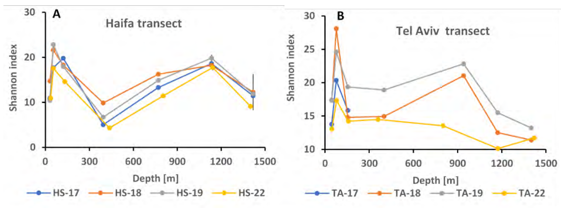
איור 4.14: מדד שאנון בניטורי הים העמוק בשנים 2017-2022. A- חתך חיפה. B- חתך תל אביב.
