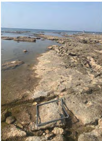
איור 6.6: איזור גב הטבלה בשקמונה בו נעשו הדיגומים (פאנל שמאלי) וצלחית מיובשת ומתה ליד ה"צלקת" שלה (פאנל ימני).
