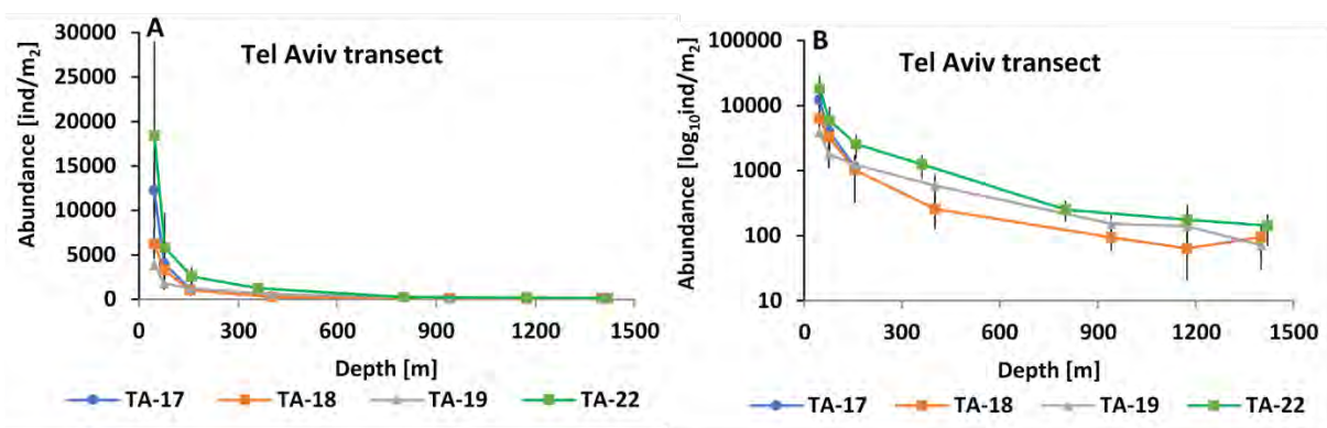
איור 4.12: צפיפות חי תוך המצע, חתך תל אביב, בניטורי הים העמוק בשנים 2017-2022. A- סקאלה לינארית. B- סקאלה לוגריתמית.
