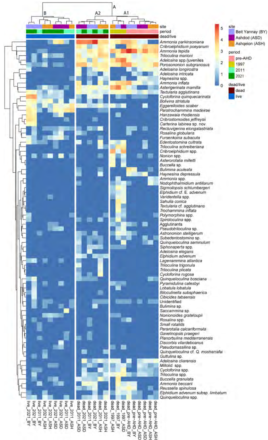
איור 4.15: אנליזת מקבצים - Q-mode Ward.D hierarchical cluster analysis - הכוללת דוגמאות פני שטח ותת הקרקע בשלוש תחנות בית ינאי (BY), אשקלון (ASH) ואשדוד (ASD) בדרום מזרח הים התיכון המייצגות ארבע פרסות זמן- טרוס סכירת הנילוס, 1997 (Hyams-) 2011 (Kaphzan et al. 2008), 2021 (Avnaim-Katav et al., 2020) ו-2021. האנליזה כללה 101 מינים המייצגים >2% מסך מאסף הפורמיניפרים
