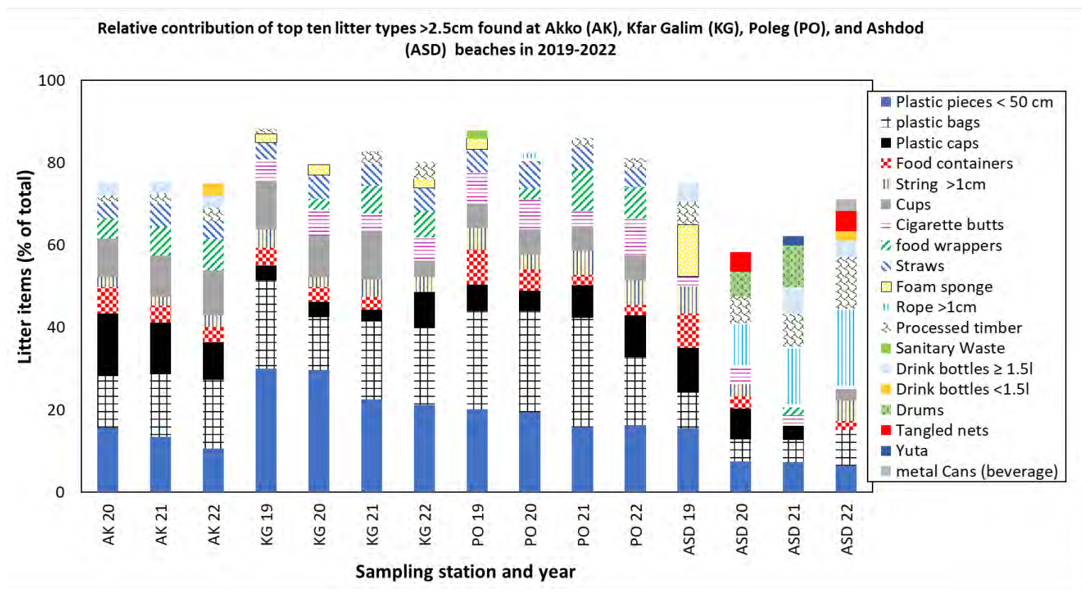
איור 3.3: עשרת הפרטים הנפוצים שנאספו בחופי עכו (AK), כפר גלים (KG), פולג (PO) ואשדוד (ASD) בשנים 2019-2022.
