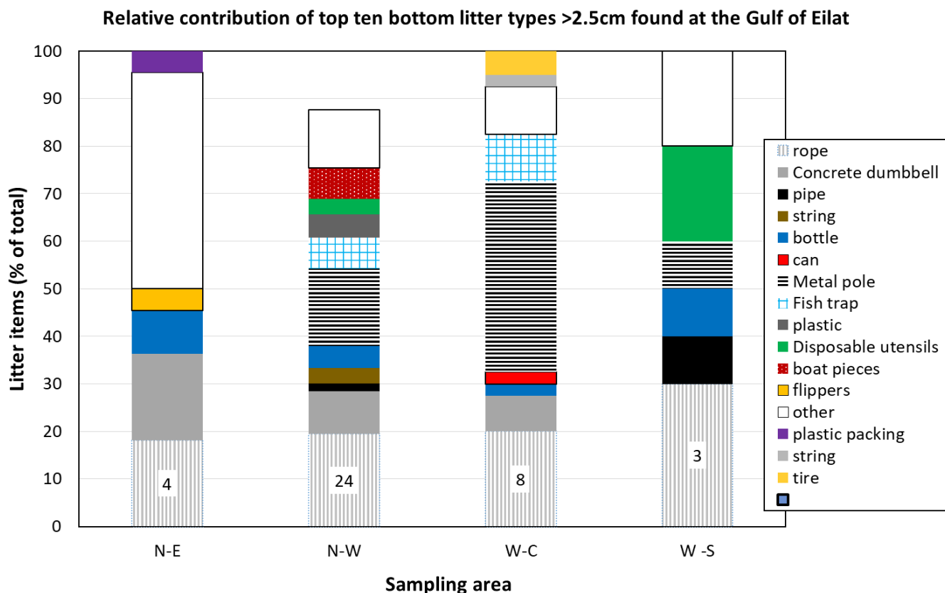
איור 6.2 עשרת הפרטים הנפוצים בפסולת הקרקעית באילת בשנת 2022, בחלוקה על פי אזורי הדיגום. המספר בעמודת החבלים מייצגת את כמות החבלים שנצפו.
