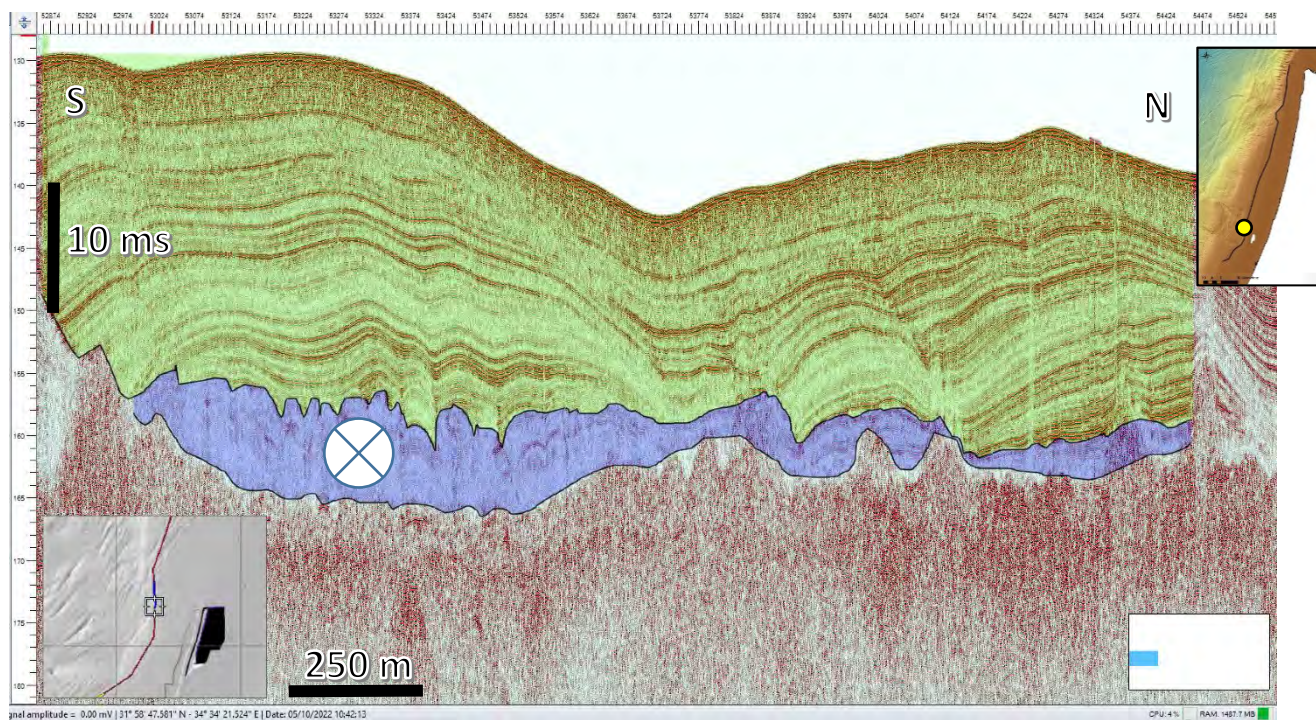
איור 14: דוגמא לגלישה בדרום מול פלמחים, ליד הצלקת המזרחית של גלישת פלמחים. היחידה הסגולה מפוענחת כיחידה שגלישה ויושבת באי התאמה מעל היחידה שמתחתיה ומעליה. מהחתך נראה שהיחידה הירוקה שקעה לאחר מכן. עומק המים הוא כ- 90 מ'. הסימון על היחידה הסגולה מציין תנועה בכיוון אל תוך הדף (בכיוון מערב).
