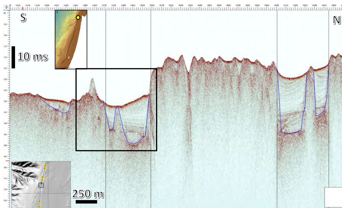
איור 15: דוגמא לראש-קביון קבור בתת-הקרקע. האופק הסגול היושב באי-התאמה ליחידה שמתחתיו מפוענח כחלקו התחתון של הקביון הנמשך מערבה (לתוך הדף). עומק המים כ- 75-90 מ'. חלק החתך המוצג באיור הבא מסומן בשחור.
