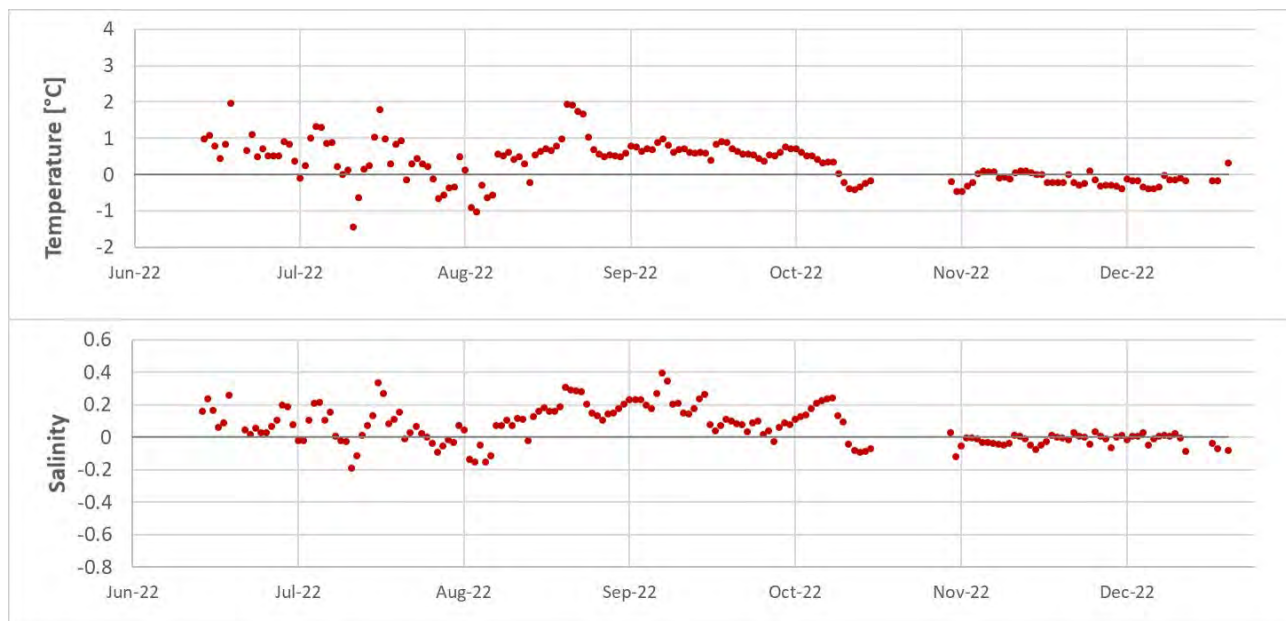
איור 1.11: השוואת ממוצעים יומיים של טמפרטורה ומליחות הנמדדים בתחנות אשקלון וחדרה למחצית השנייה של שנת 2022 (מאז חידוש המדידות באשקלון). הערכים המוצגים הינם השארית לאחר חיסור הערך הנמדד בתחנת חדרה מזה הנמדד בתחנת אשקלון.
