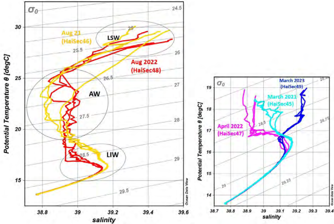
איור 1.5: דיאגרמות \theta/S של תצפיות בתחנות H04, H05 ו-H06 במרץ 2021, אפריל 2022 ומרץ 2023 (ימין), ובאוגוסט 2021 ו-2022 (שמאל). זיהוי מסות מים אופייניות מסומן בדיאגרמה הקיצית.
