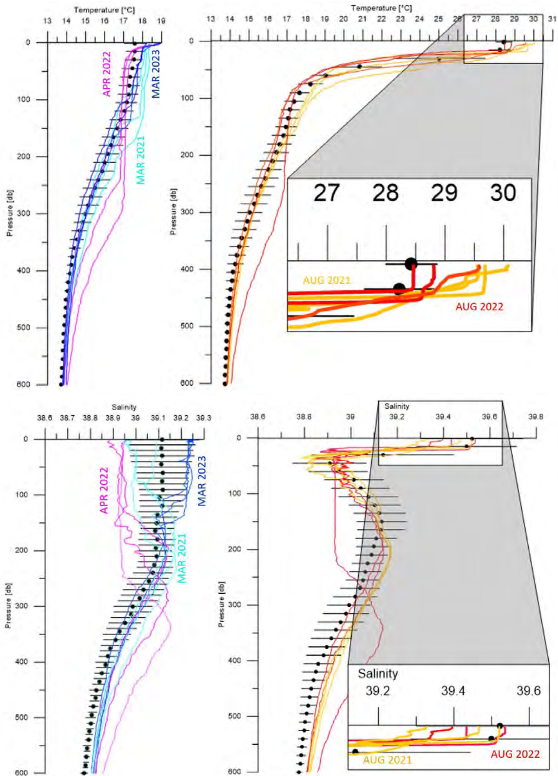
איור 1.4: פרופיל טמפרטורה (למעלה) ומליחות (למטה) בתחנות H04, H05, ו- H06 במרץ 2023 ובאפריל 2022 (שמאל) ובאוגוסט 2021 ו-2022 (ימין). ממוצעים עונתיים כפי שחשבו ממדידות בתחנות H05 ו-H06 מוצגים כנקודות שחורות עם קווי שגיאה.
