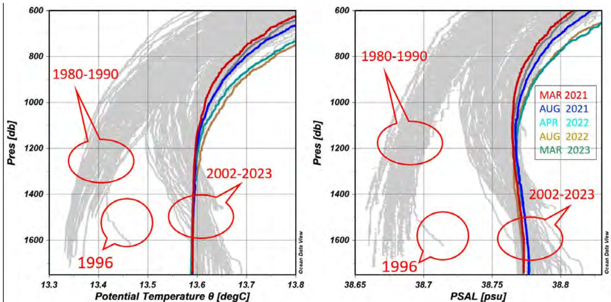
איור 1.6: שינויים רב-שנתיים בטמפרטורה פוטנציאלית ומליחות מי העומק במזרח הים התיכון כפי שנצפו בפרופילים האנכיים בתחנות H05 ו-H06. בפרופיל מ-1996 ניתן לראות את הגעת מסת מים שמקורה באנומליית האיגאי למדרון מדף היבשת הישראלי. פרופילים בצבע – המדידות בשנים 2021-2023.
