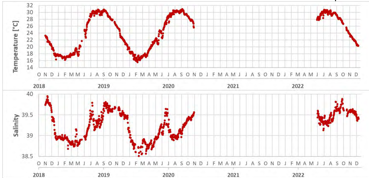
איור 1.9: ממוצעים יומיים של טמפרטורה ומליחות הנמדדים בתחנת חדרה באמצעות מכשיר CTD לתקופה פברואר 2014 ועד ינואר 2023.
