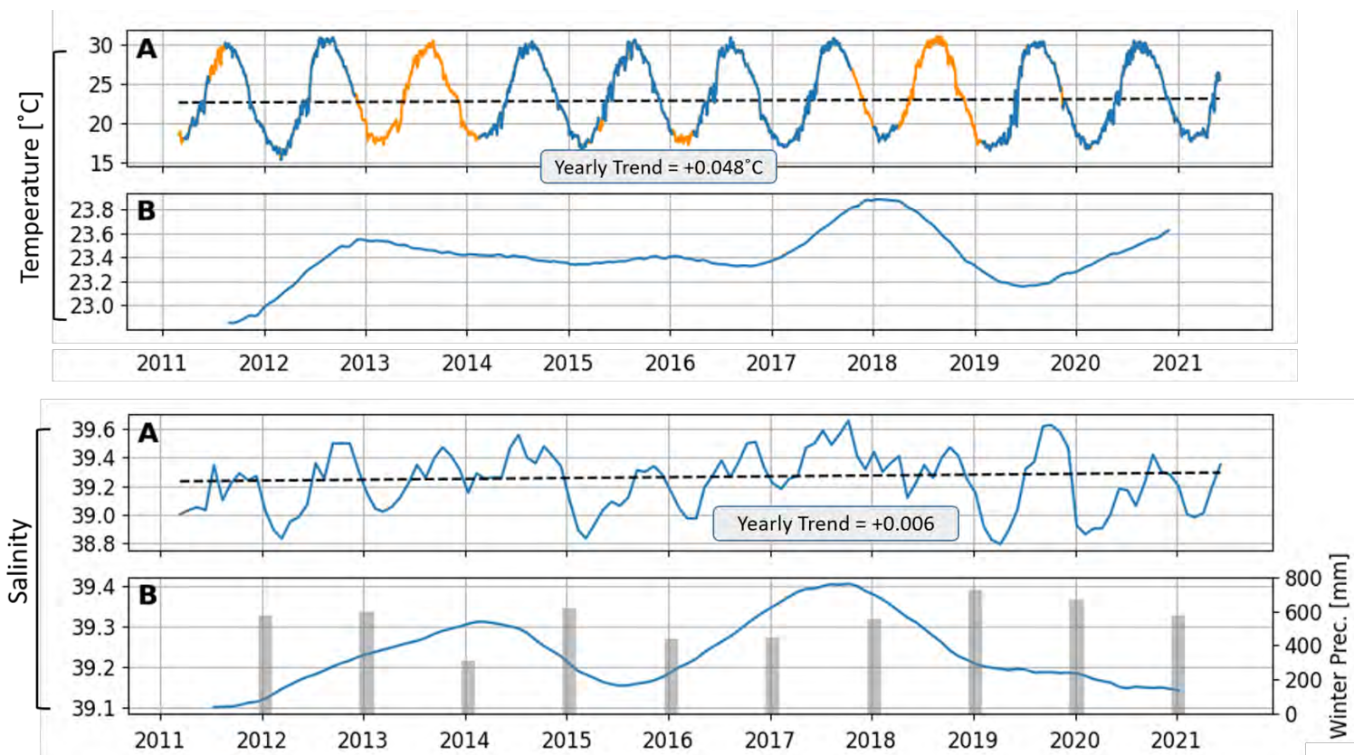
איור 1.14: סדרות זמן של טמפרטורה ומליחות עם חישוב מגמת שינוי שנתי בשטח (A) Mann-Kendall test. ניתוח של מגמות רב שנתיות על ידי דיקומפוזיציה של סדרת הזמן בשטח X11-ARIMA (B). משקעים שנתיים (ערך מצטבר לכל עונת חורף) מוצגים גל גבי סדרת המליחות באפור.
